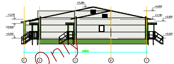
Facade E-A
