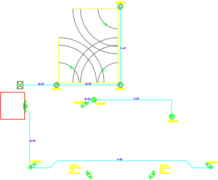
PLANTA DE DISTRIBUCI?N DE SISTEMA DE CCTV NIVEL 1 CDI – CLUB DE PLAYA EL BALSAMAR Esc 1:75
