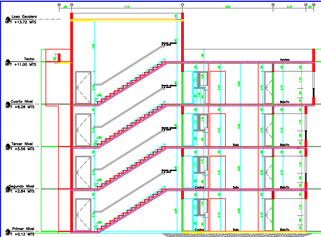
Secci?n Longitudinal Z-Z' Tipo I Esc. 1:50
