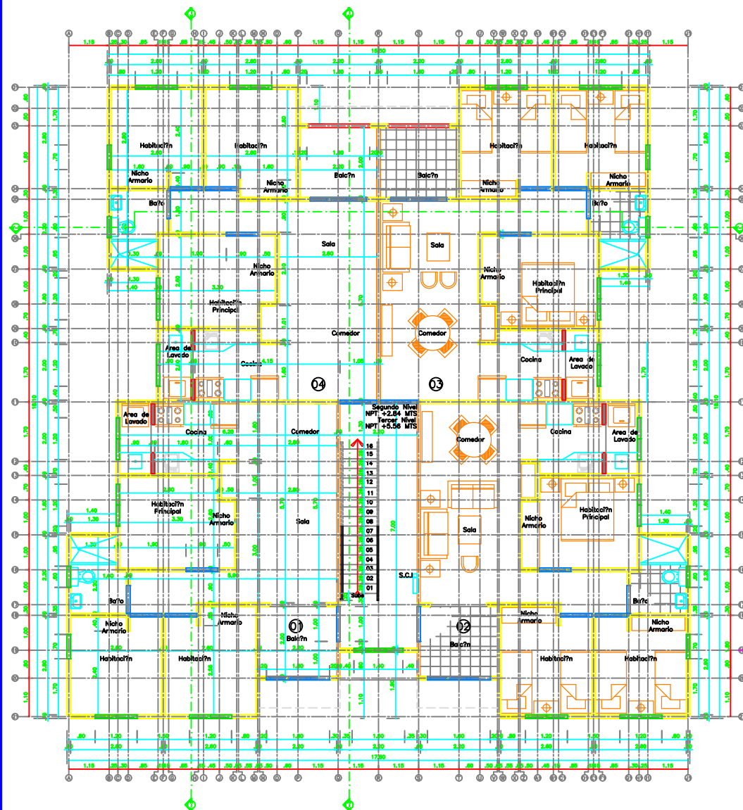
Planta Arquitect?nica Tipo I 4to. Nivel Esc. 1:50
