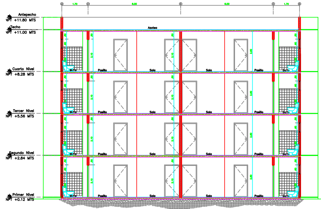
Sección Transversal Y-Y' Tipo I Esc. 1:50
