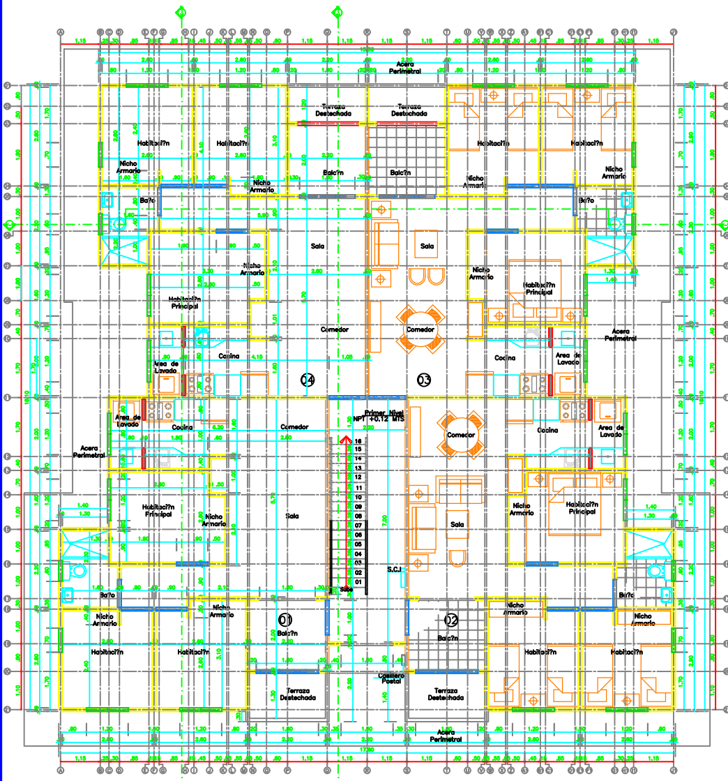
Planta Arquitectónica Tipo I 1er. Nivel Esc. 1:50
