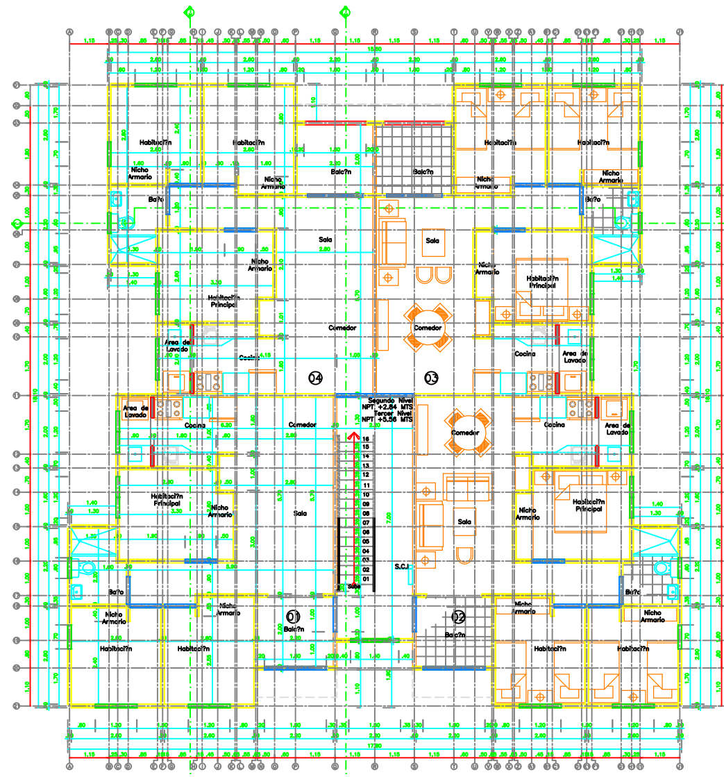
Planta Arquitectónica Tipo I 2do. y 3er. Nivel Esc. 1:50
