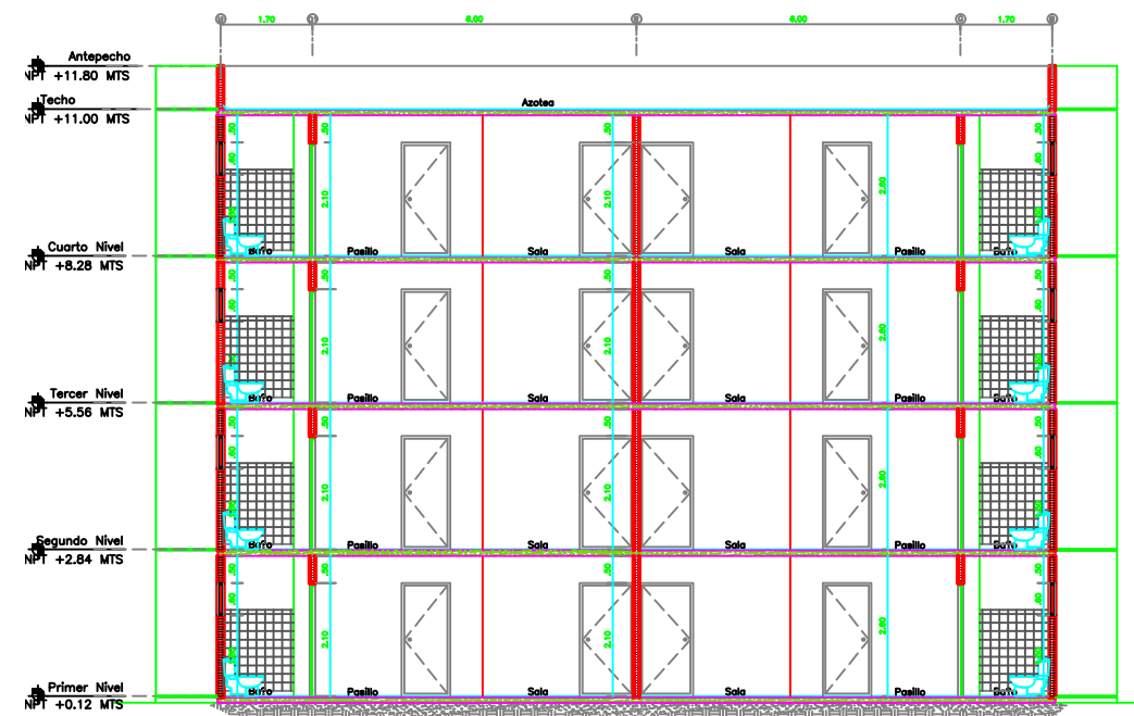
Secci?n Transversal Y-Y' Tipo I Esc. 1:50
